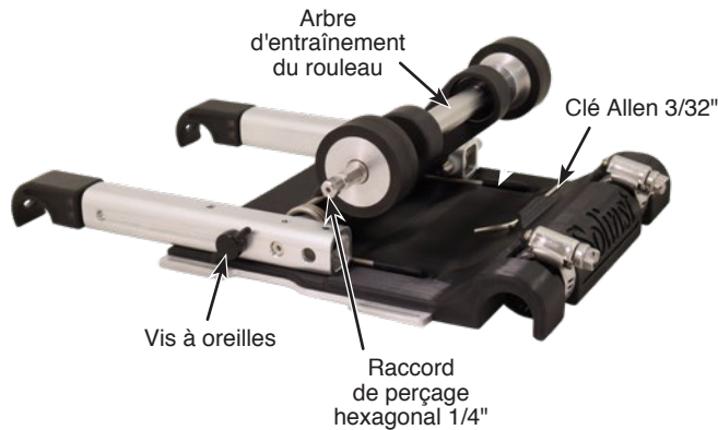
Enrouleur Solinst Modèle 101 (#116159)
