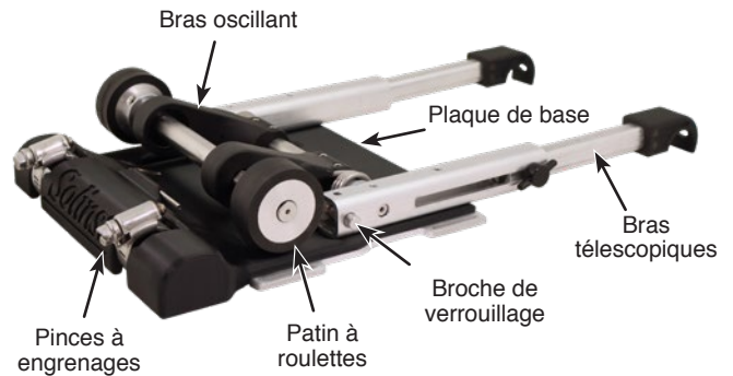
Enrouleur Solinst Modèle 101 (#116159)
